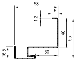
OSMK door frame profile
