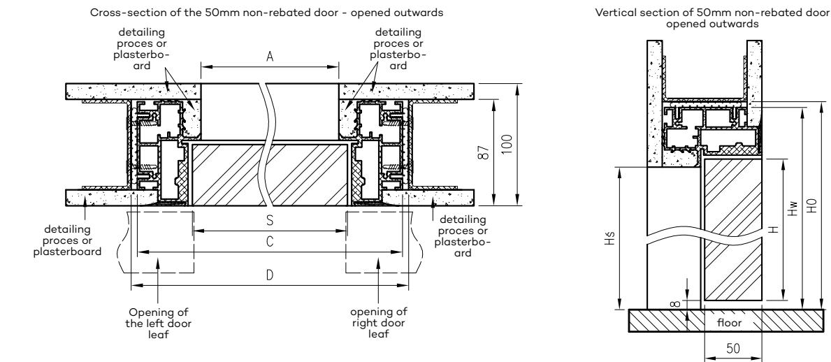
Profi door width dimensions
