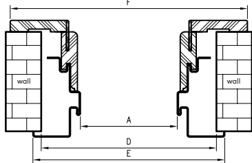
door frame profile
