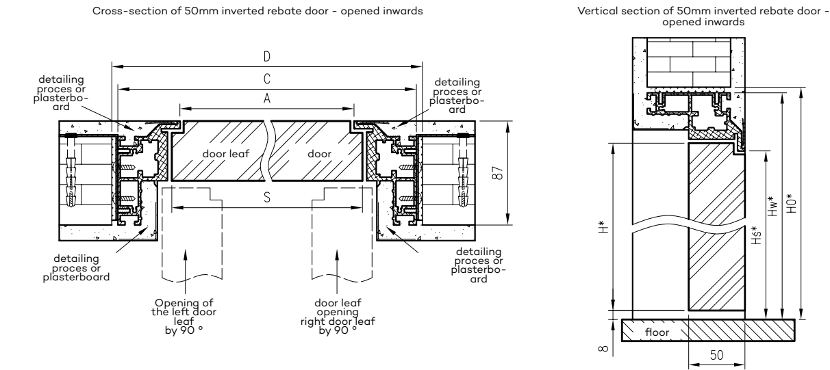
Profi door width dimensions
